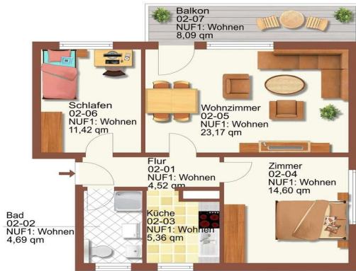
Obergeschoss rechts
